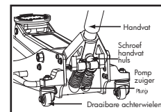
Achterkant van de krik
