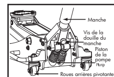
Arrière du cric
