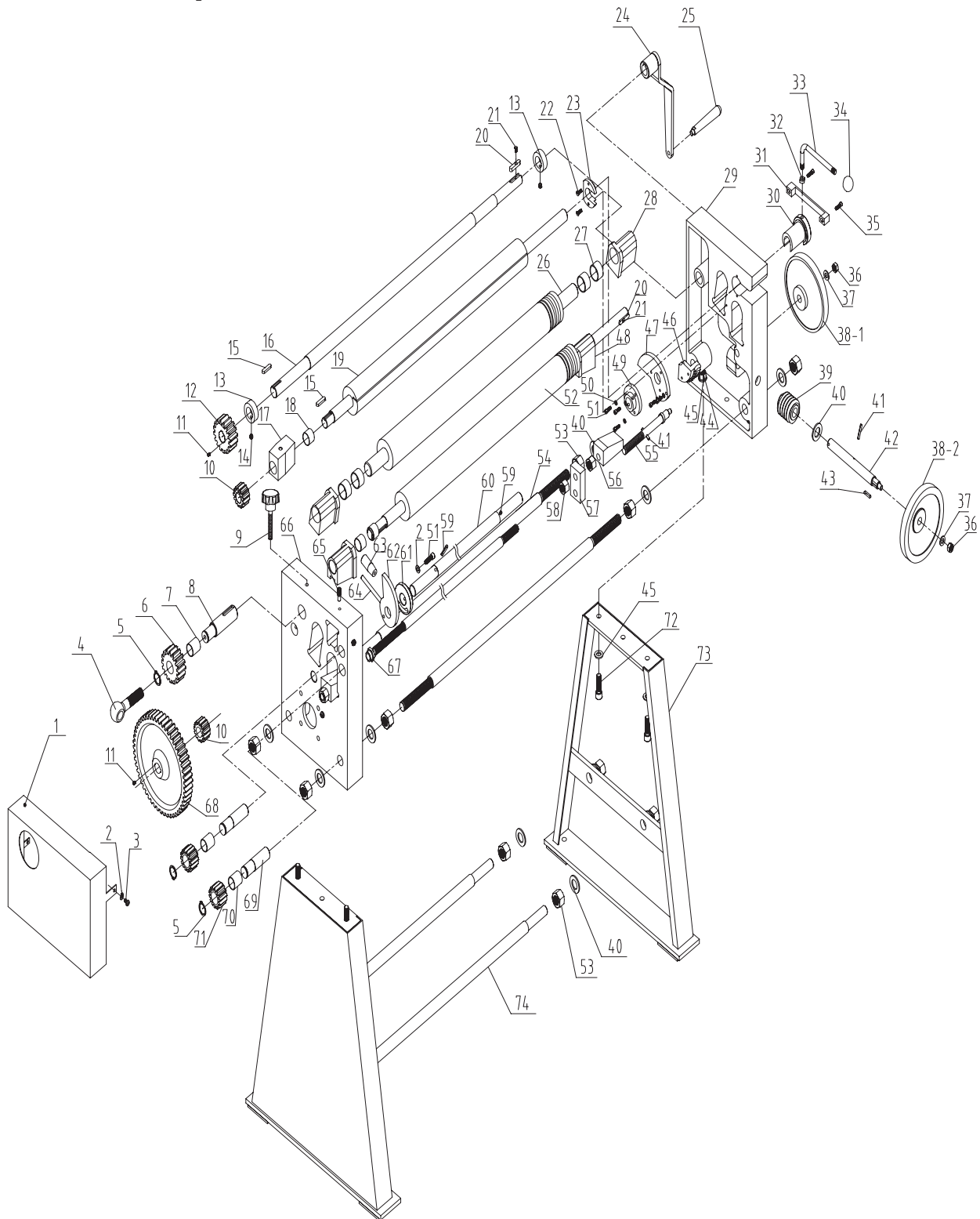
Fig. 5-1: Dessin des pièces détachées
