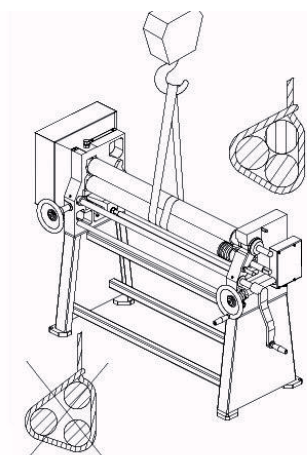
Fig. 3-1: Montage
